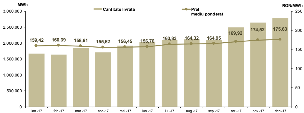
Figura 4: Evoluția livrărilor de energie electrică prevăzute în contractele încheiate pe PCCB – modalitatea de tranzaționare PCCB-LE și prețul mediu corespunzător acestora
