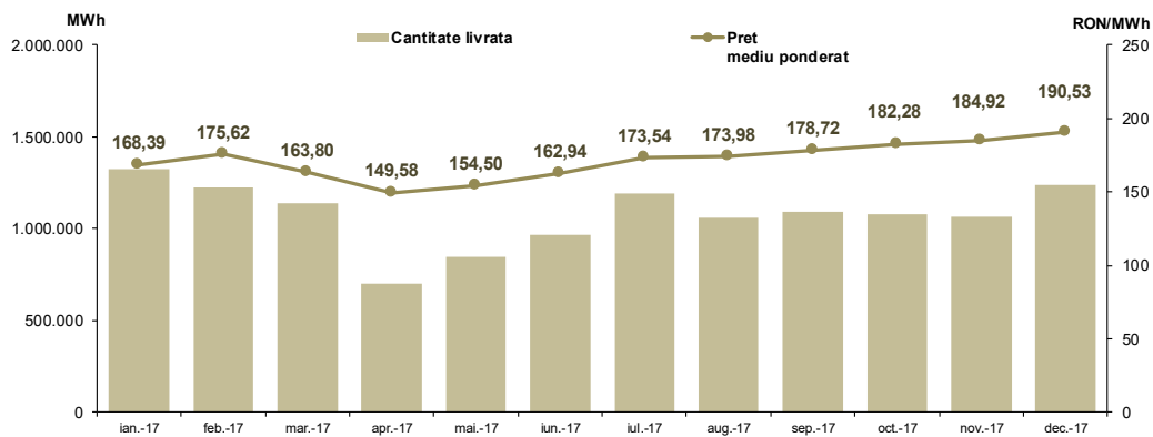
Figura 5: Evoluția livrărilor de energie electrică prevăzute în contractele încheiate pe PCCB – modalitatea de tranzaționare PCCB-NC și prețul mediu corespunzător acestora
