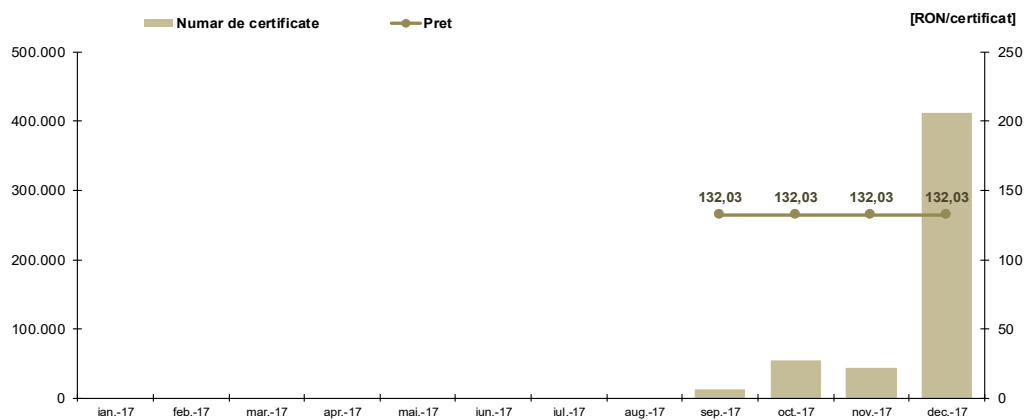
Figura 9: Evoluția prețului și numărului de certificate verzi tranzacționate pe PCSCV
